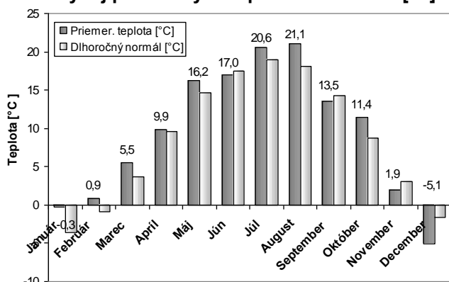
Vývoj priemerných teplôt v roku 2001 [°C]
