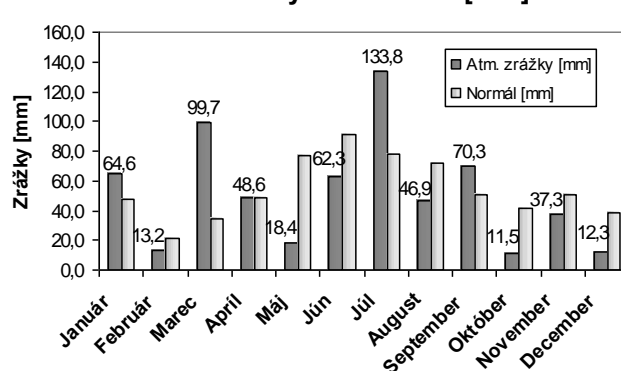
Atm.zrážky v roku 2001 [mm]
