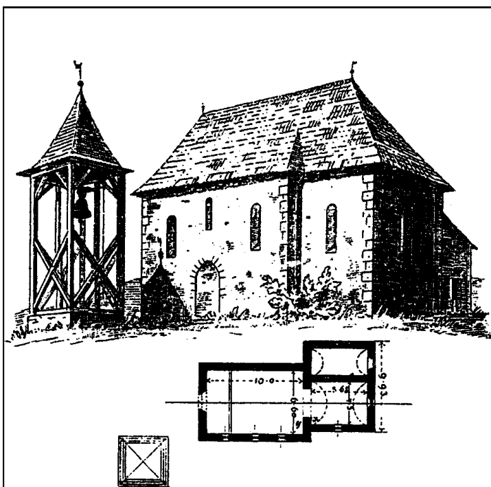
A CSÉCSI TEMPLOM LÁTKÉPE ÉS ALAPRAJZA.
